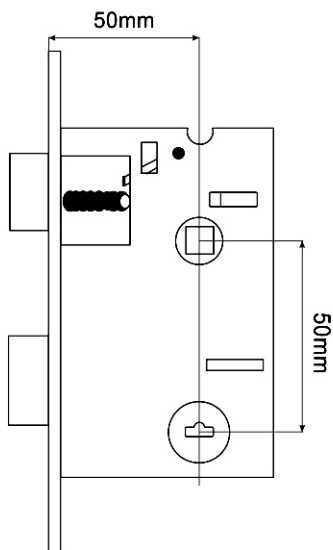
Модель механизма (50 50) 22 x 160mm
