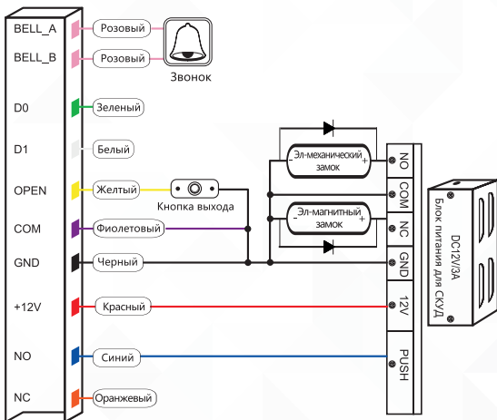
Типовая схема подключения в режиме автономного контроллера (блок питания для систем контроля доступа)
