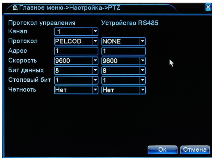
Рис. 4.3.6. Настройка. PTZ
