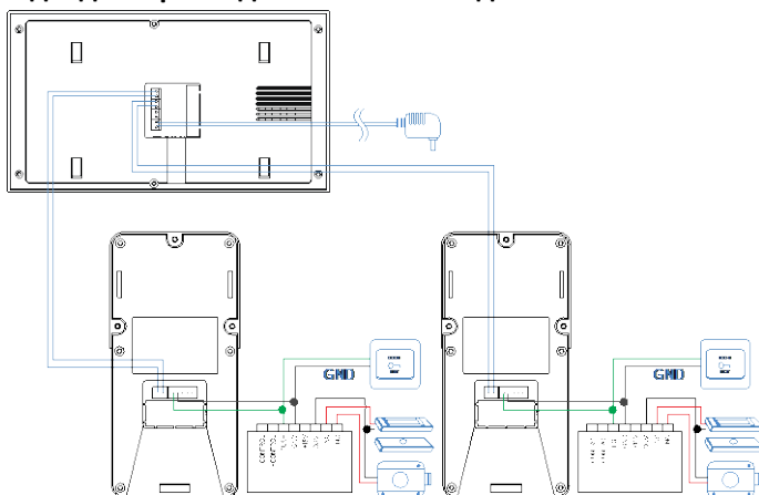
Изображение 1-8 Схема подключения питания системы контроля доступа. Один видеодомофон и две вызывных видеопанели.
